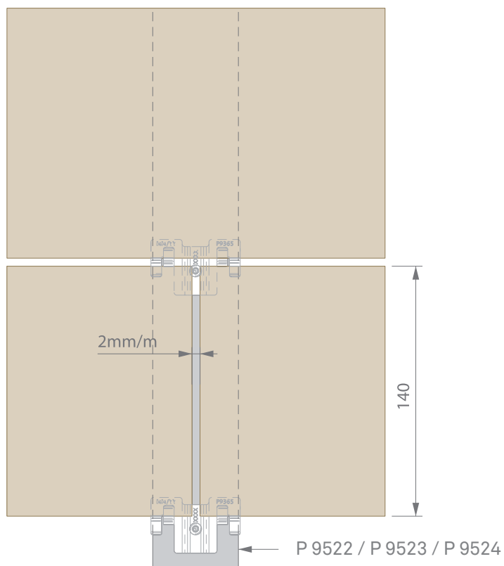
POHLED SHORA
